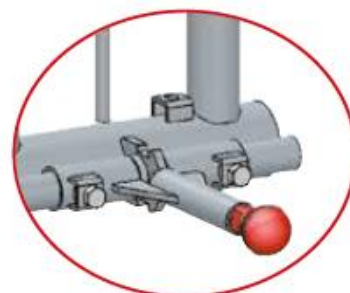
Vergrendeling door kwartslagdraai
