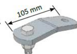
PR0298 Inclinatieplaat Voerhek - LS hek
