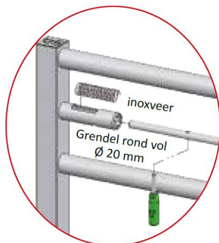
Detail van de grendelmontage
