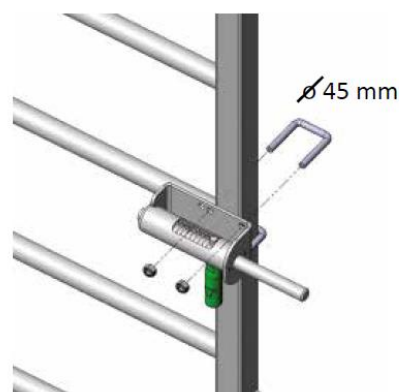
Losse grendel Autolock + draadbeugels Ø 45 mm
