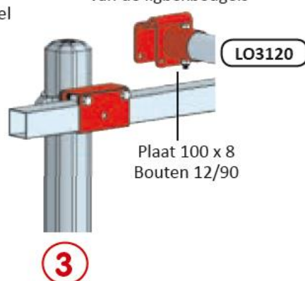
Snelle montage van de ligboxbeugels
