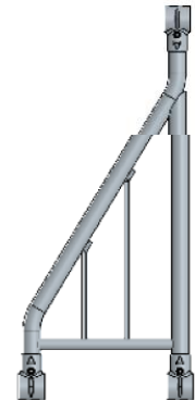
PO0419 Diagonale buis Ø 42,4 mm met anti-doorgang
