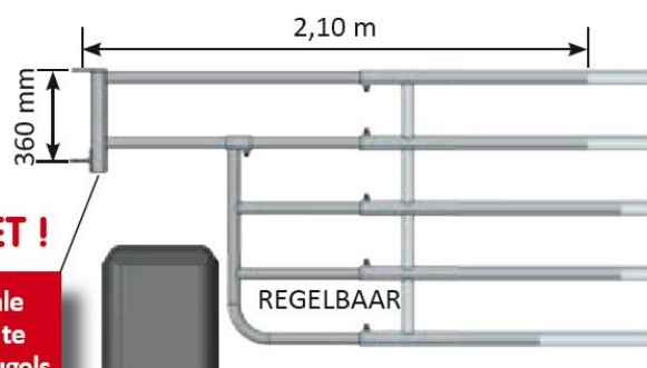
VOORKANT EX 5 voor DRINKBAK
